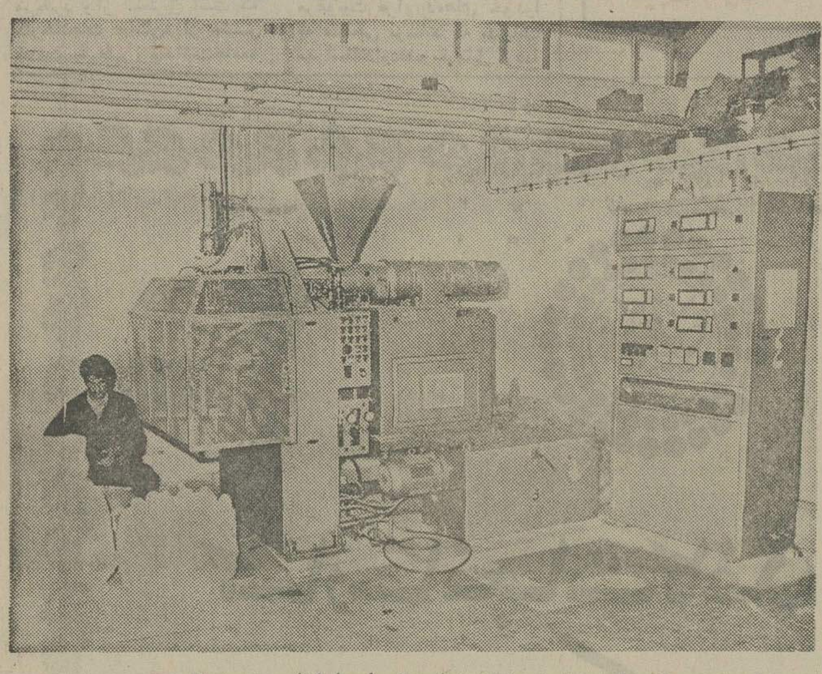
یکی از دستگاه های تمام اتوماتیک تولید ظروف پلی اتیلن برای سرکه ...
