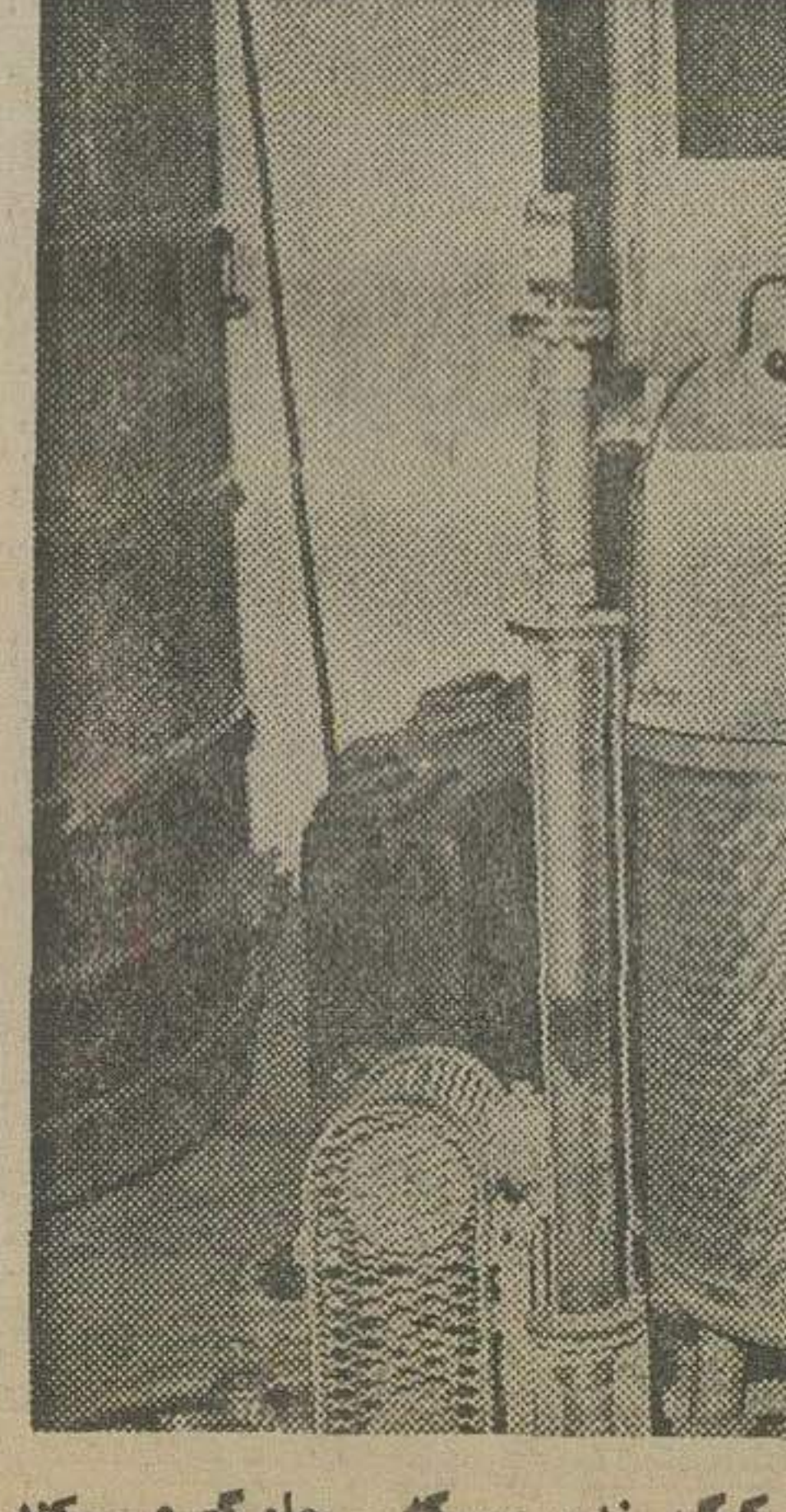
دستگاه فیلتر و پاستوریزاسیون سرکه ... این دستگاه از کبک زدن سرکه جلوگیری میکند
