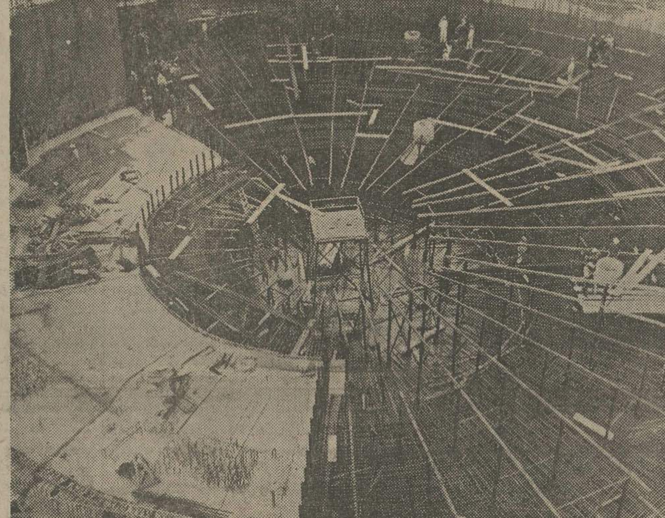
یک عکس کاملاً استثنایی - بوشهر، عملیات ساختمانی این رآکتور عظیم با تلاش شبانه روزی دهها مهندس، متخصص، کارشناس، تکنیسین و کارگر با سرعت ادامه دارد. عظمت رآکتور اتمی ایران درین عکس جالب و استثنایی، بخوبی روشن است.
