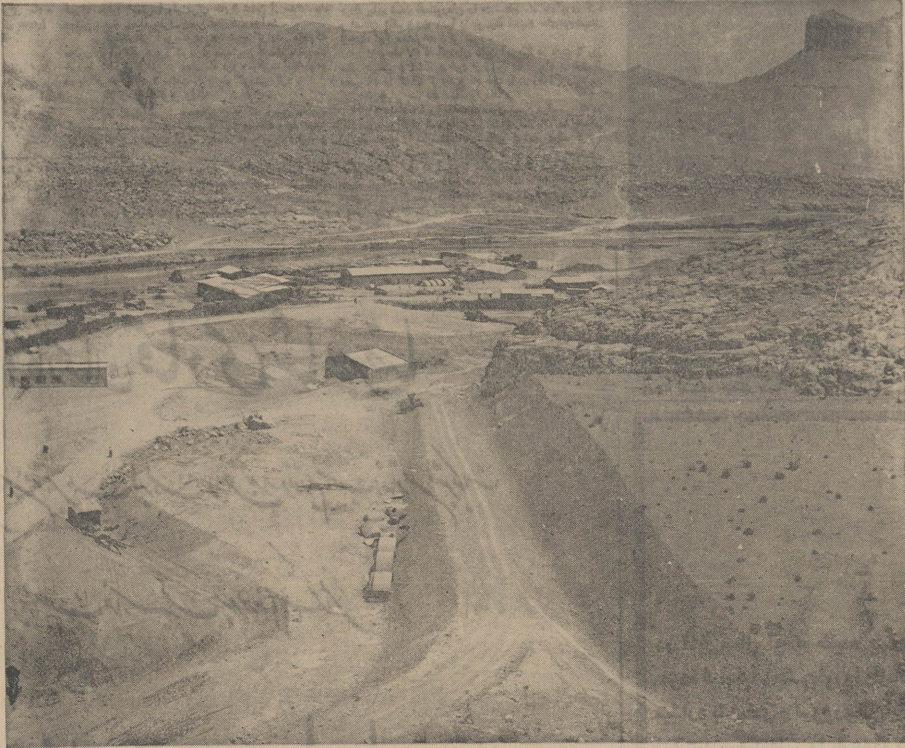
در عکس شروع کانال مشاهده میشود و در قسمت پائین عکس آخر تونل و در قسمت بالا تاسیسات مربوط به سازمان سد دیده میشود.
