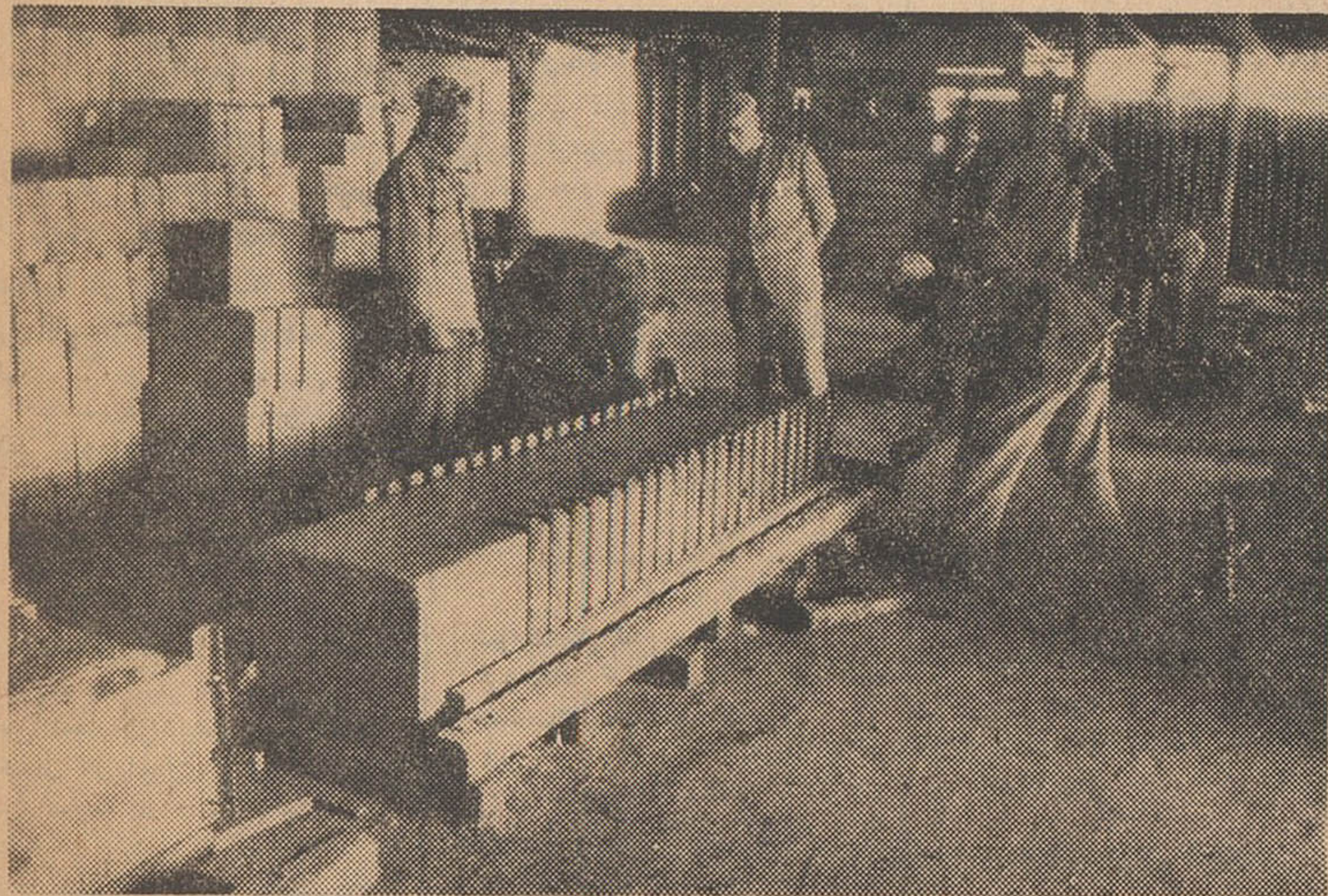
بتون‌های سبک که بوسیله متخصصین شرکت ایران راه ساخته شده است و در ساختمان فرودگاه بکاررفته است
