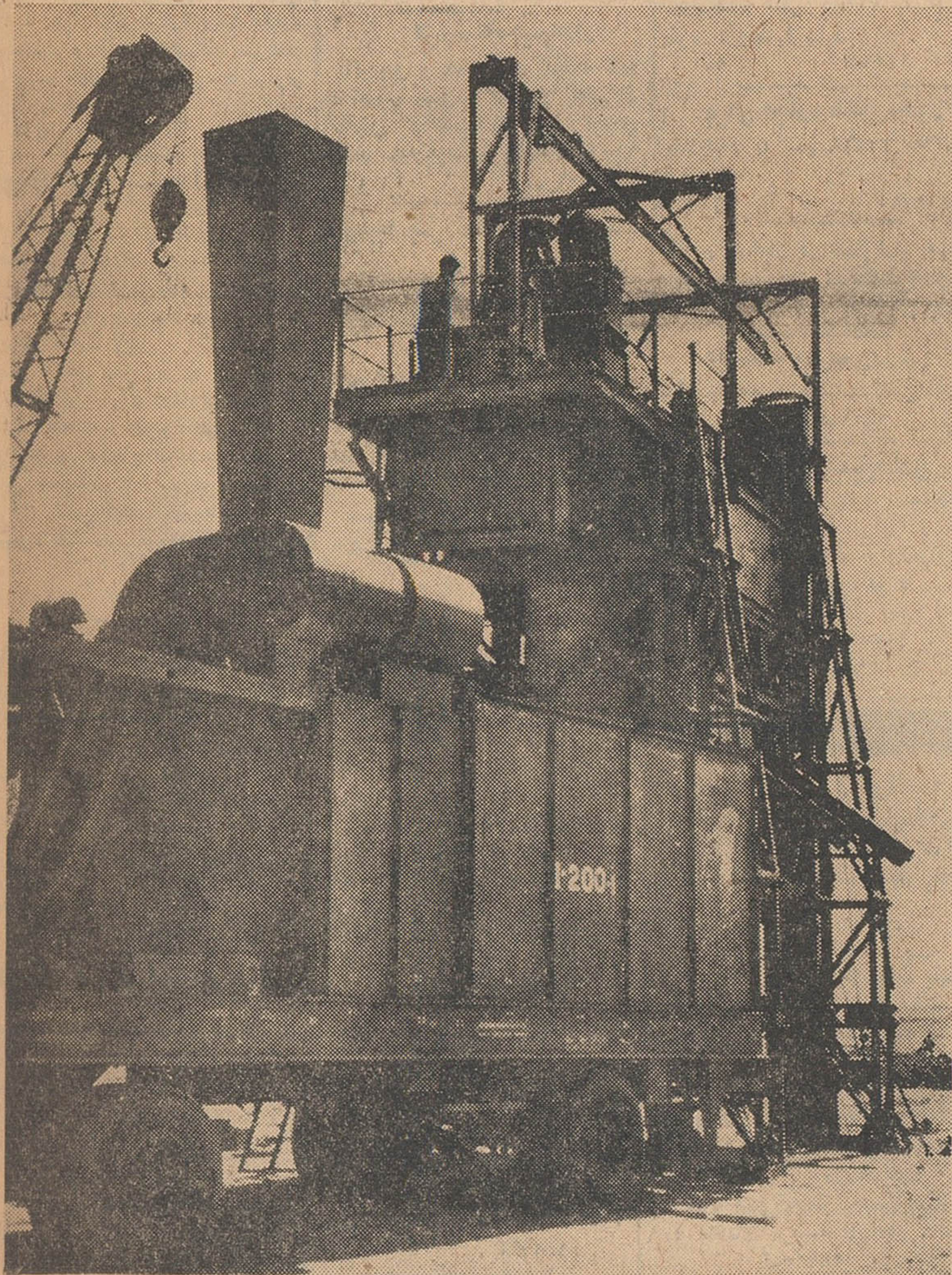
یکی از ماشین های عظیم آسفالت ریزی شرکت ایران راه که برای آسفالت باند فرودگاه شیراز بکار برده شده است
