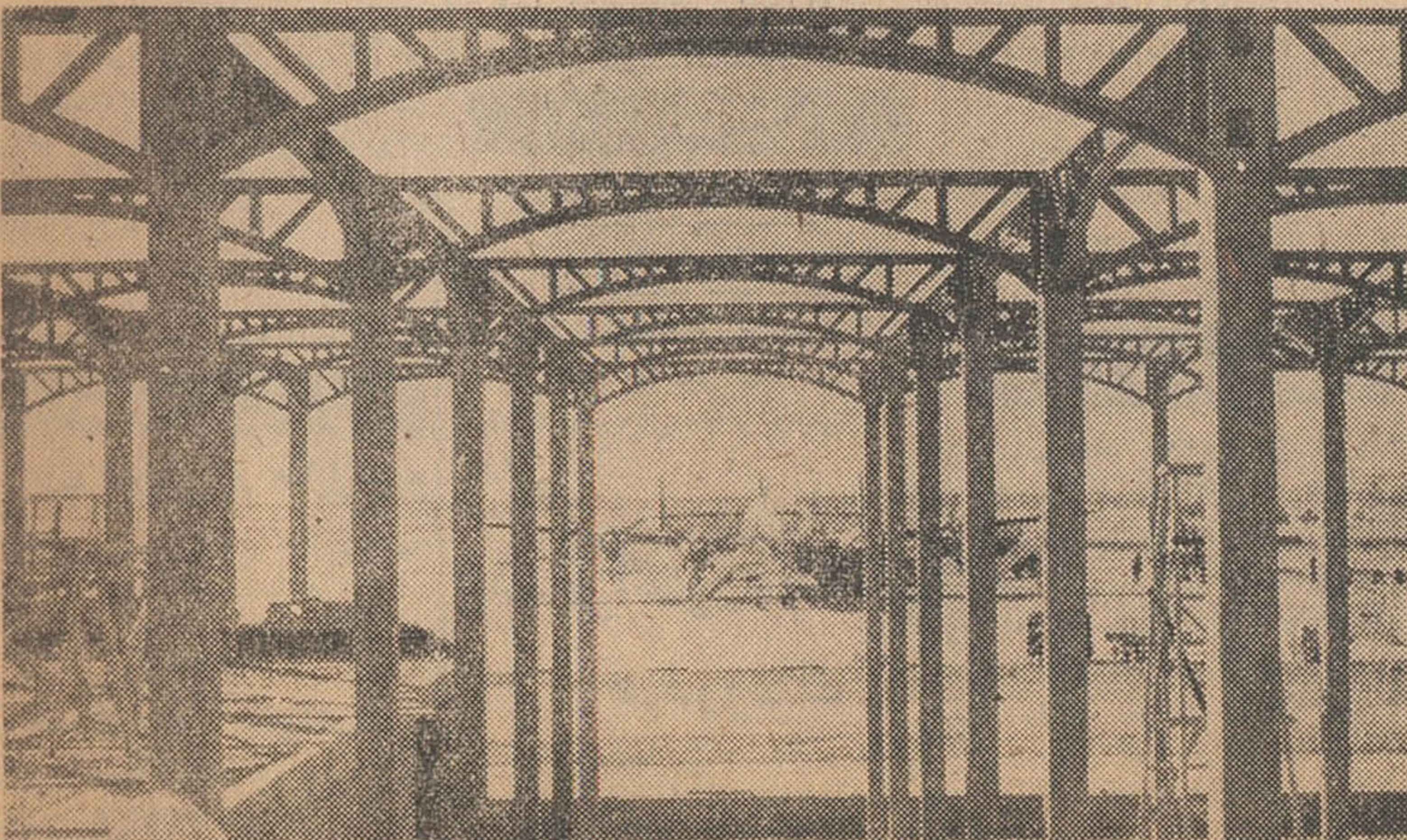
نمای اسکلت فلزی فرودگاه شیراز قبل از اتمام ساختمان
