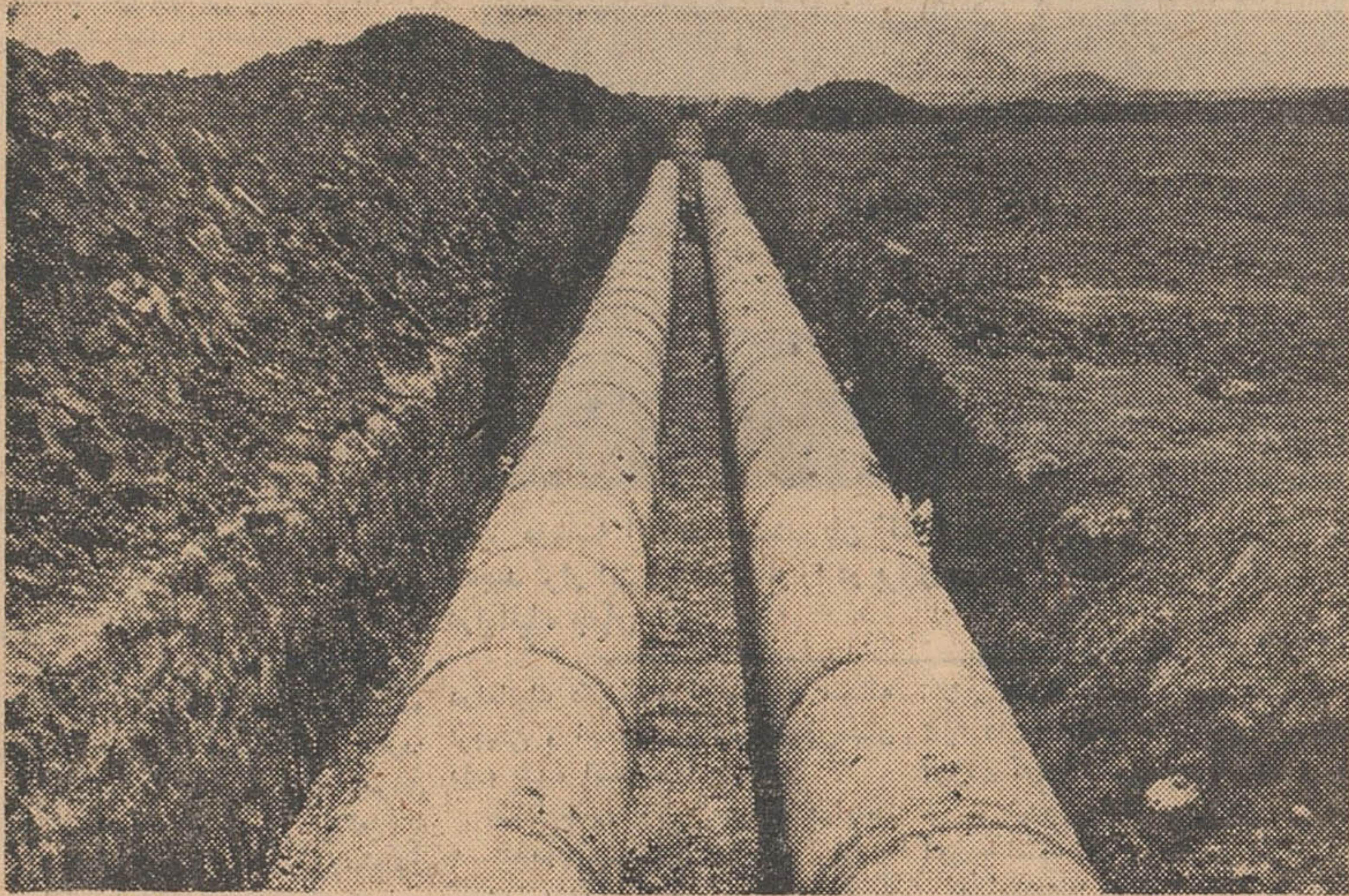
لوله های بتونی که بطول بیش از پنج هزار متر در اطراف باند و در محل های مخصوصی بکار گذارده شده است
