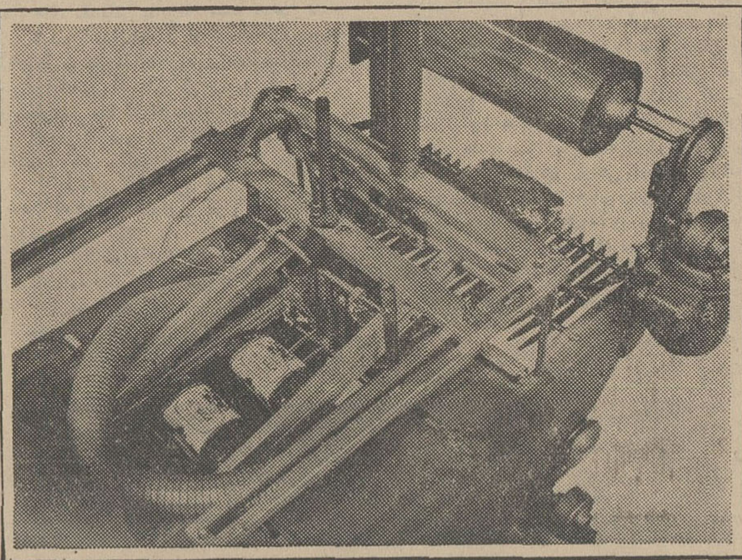
ماشین بسته بندی کتد.
