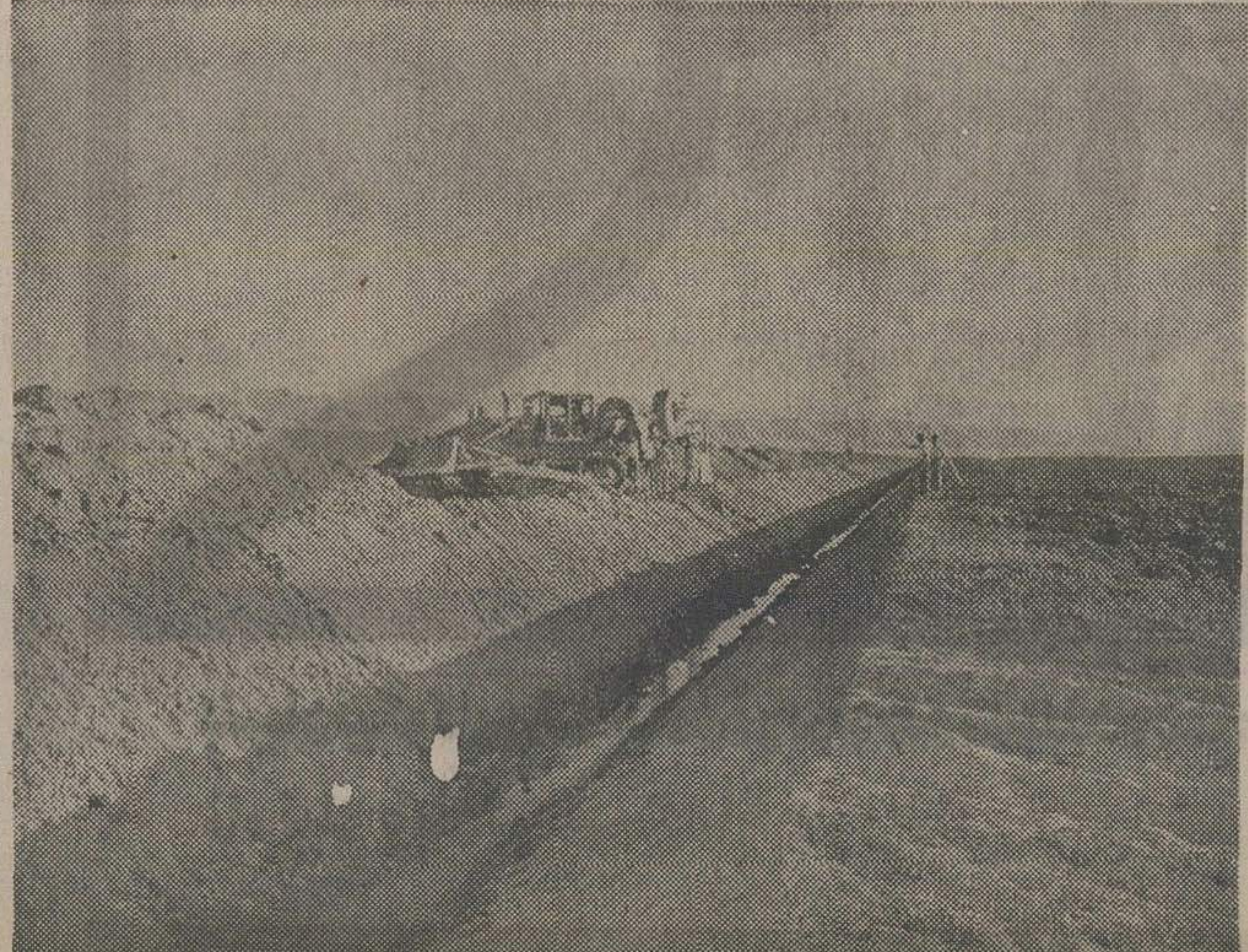
کانال خاکی انجام یافته و ماشین زهکشی که بکار مشغول است
