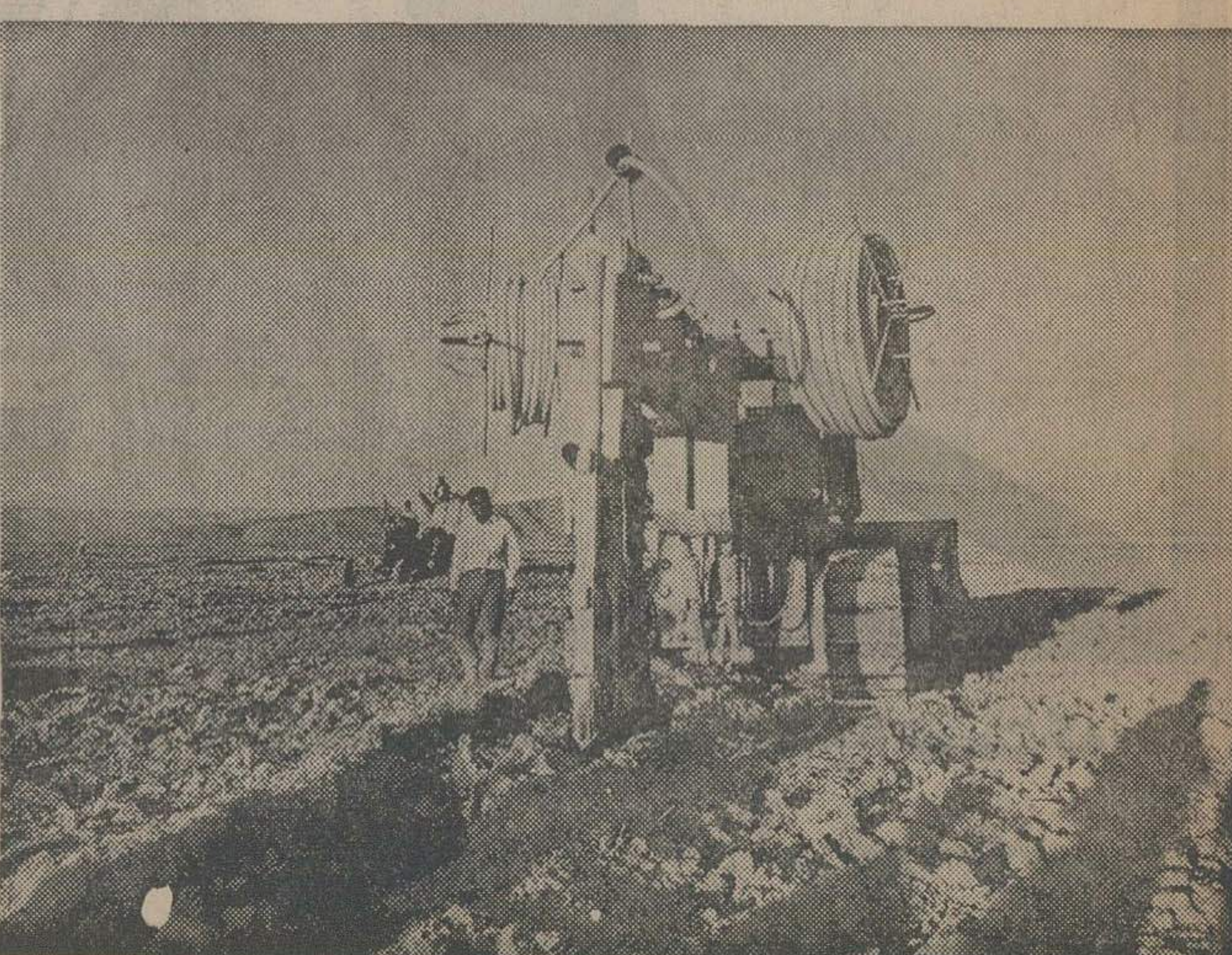
دستگاه مخصوص زهکشی در حال انجام کار
