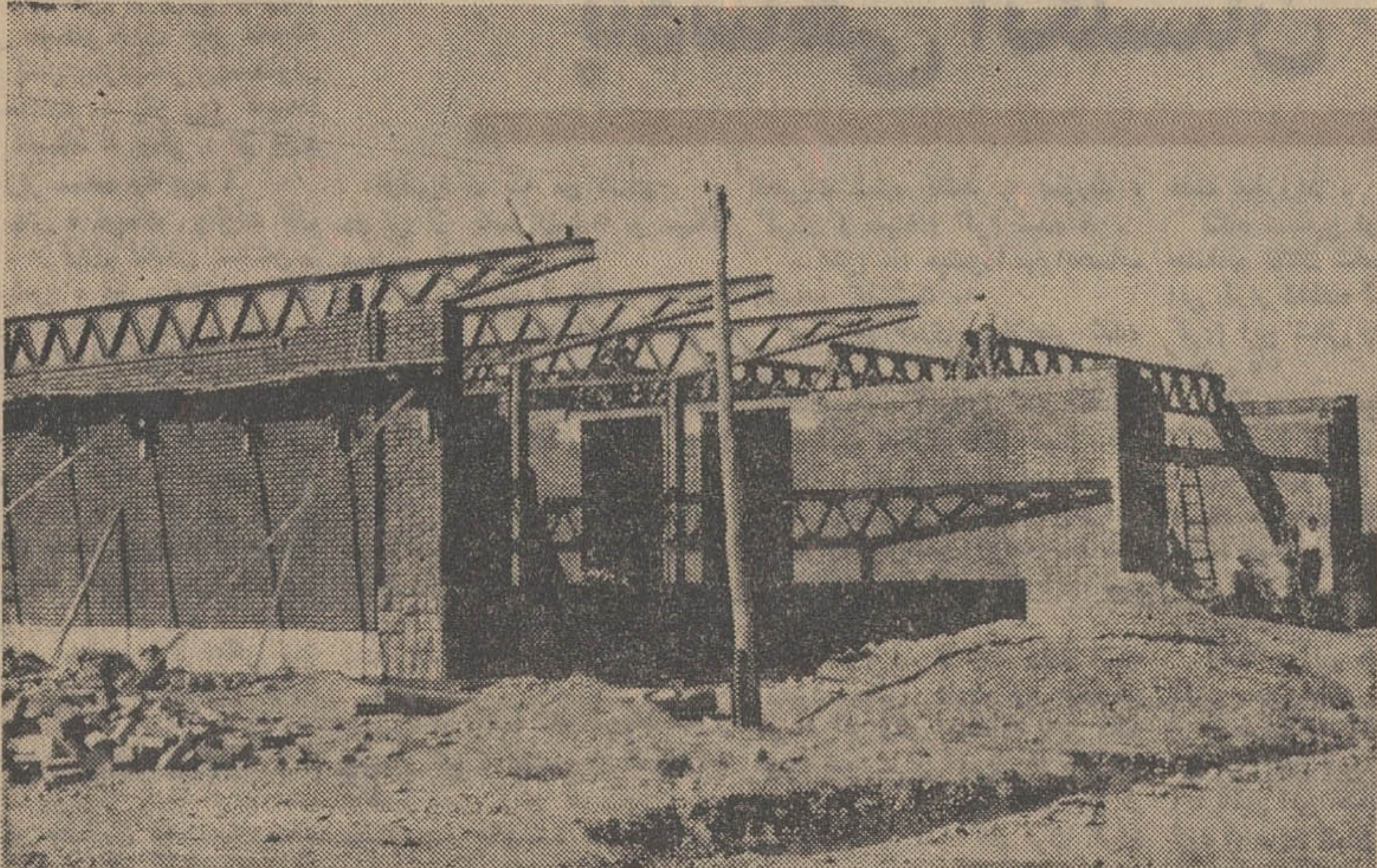
قسمتی از ساختمان کاخ جوانان رضائیه که مرحله سقف پوشی آن شروع گردیده است
