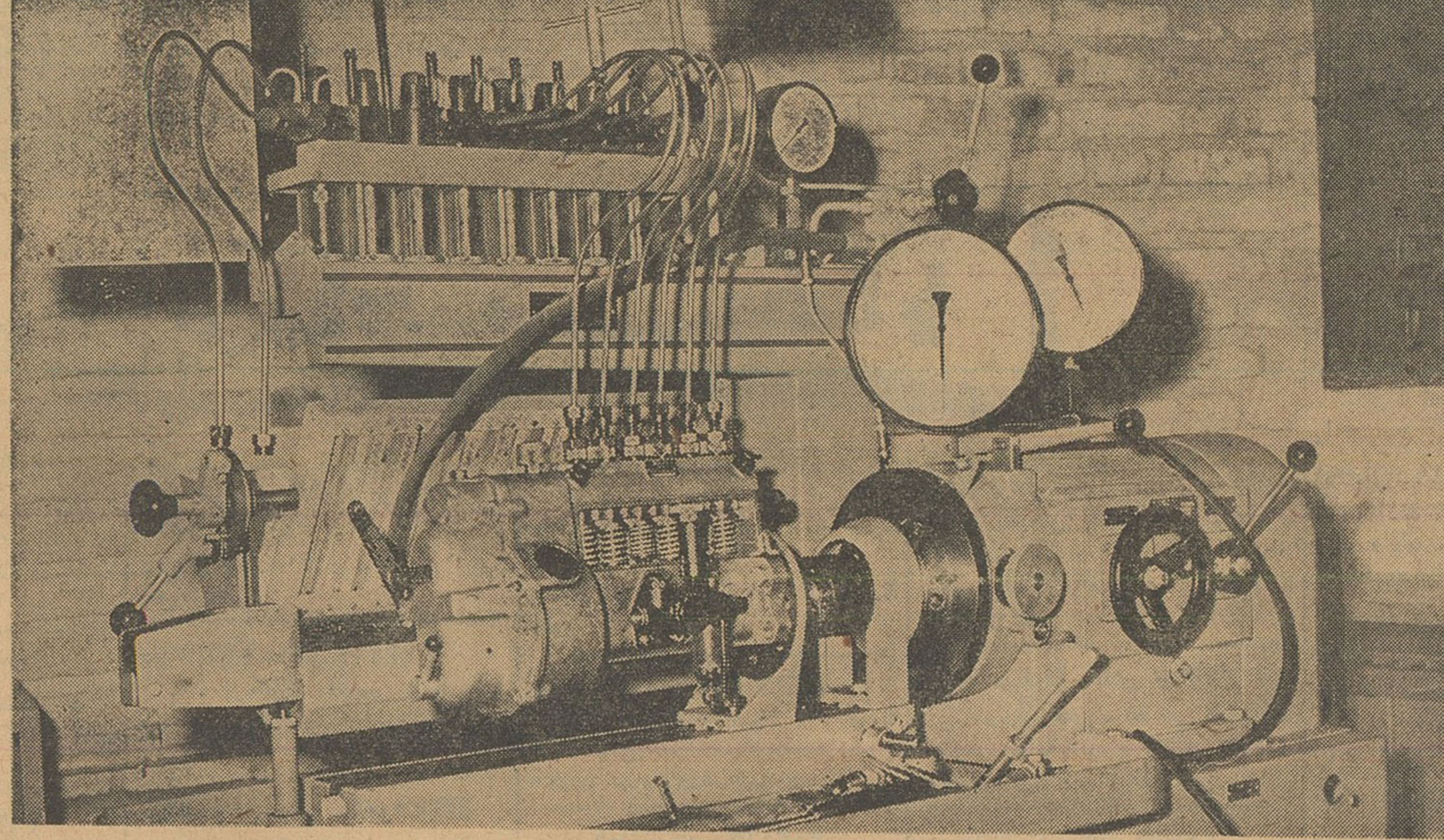
دستگاه تنظیم پمپ و فاسونکا (برای جلوگیری از دود موتورهای دیزلی) شرکت سهامی دیزل الکتریک نماینده انحصاری کارخانجات روبرت بوش آلمان در ایران
