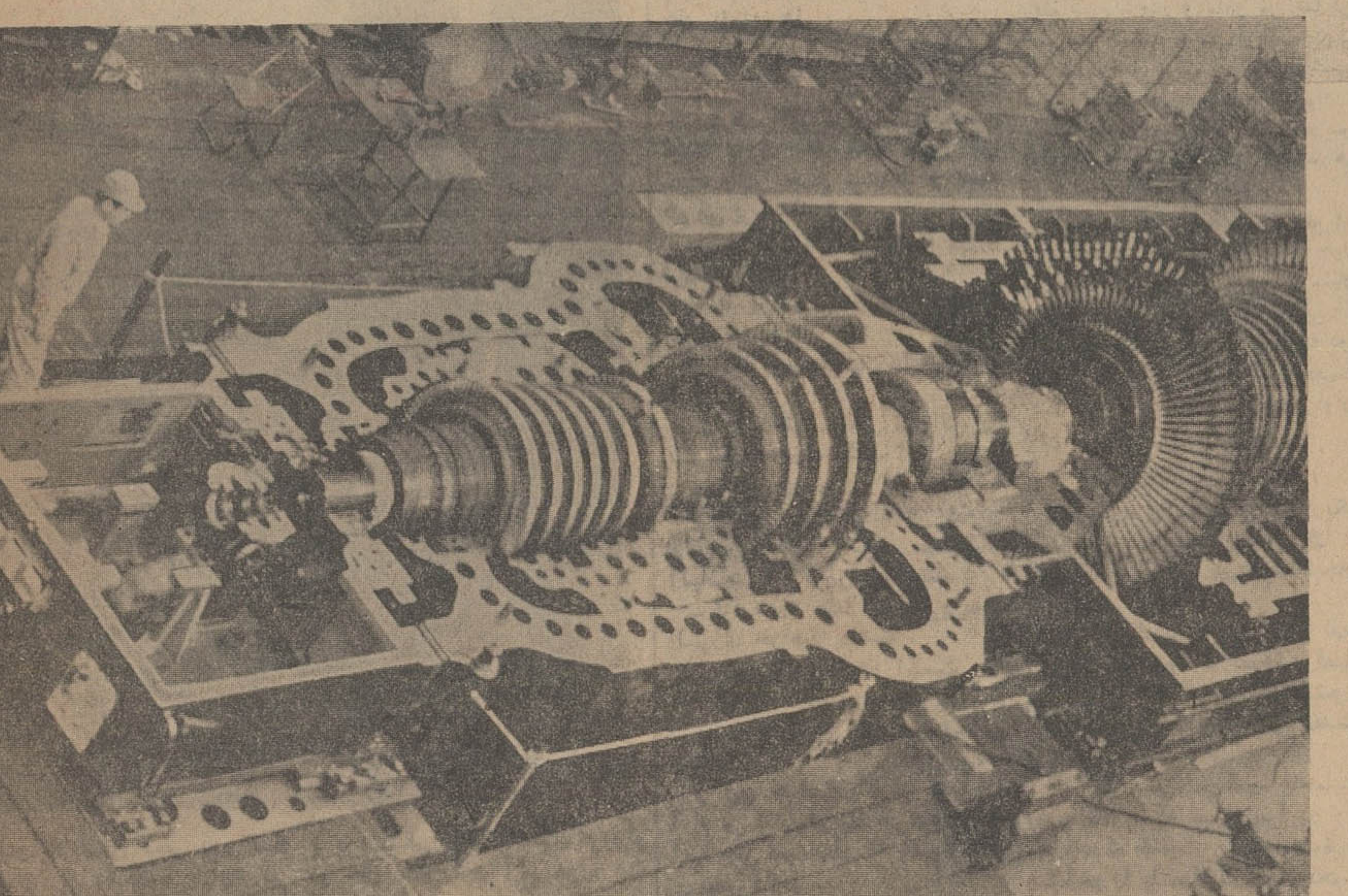
توربین ژنراتور ۳۷۵۰۰۰ کیلوواتی کارخانه برق حرارتی شهر جیتا واقع در ژاپن
