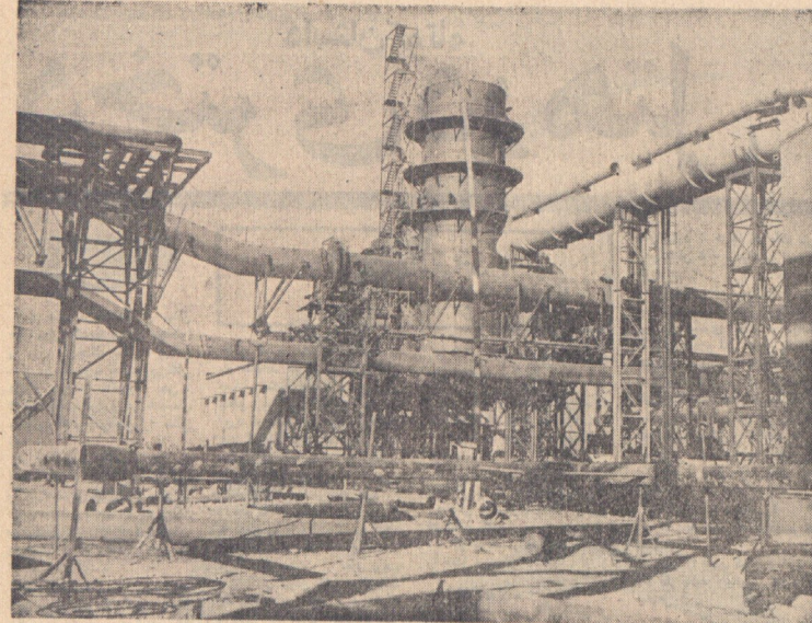
تاسیسات تصفیه گاز کوره بلند کارخانه ذوب آهن آریامهر.
