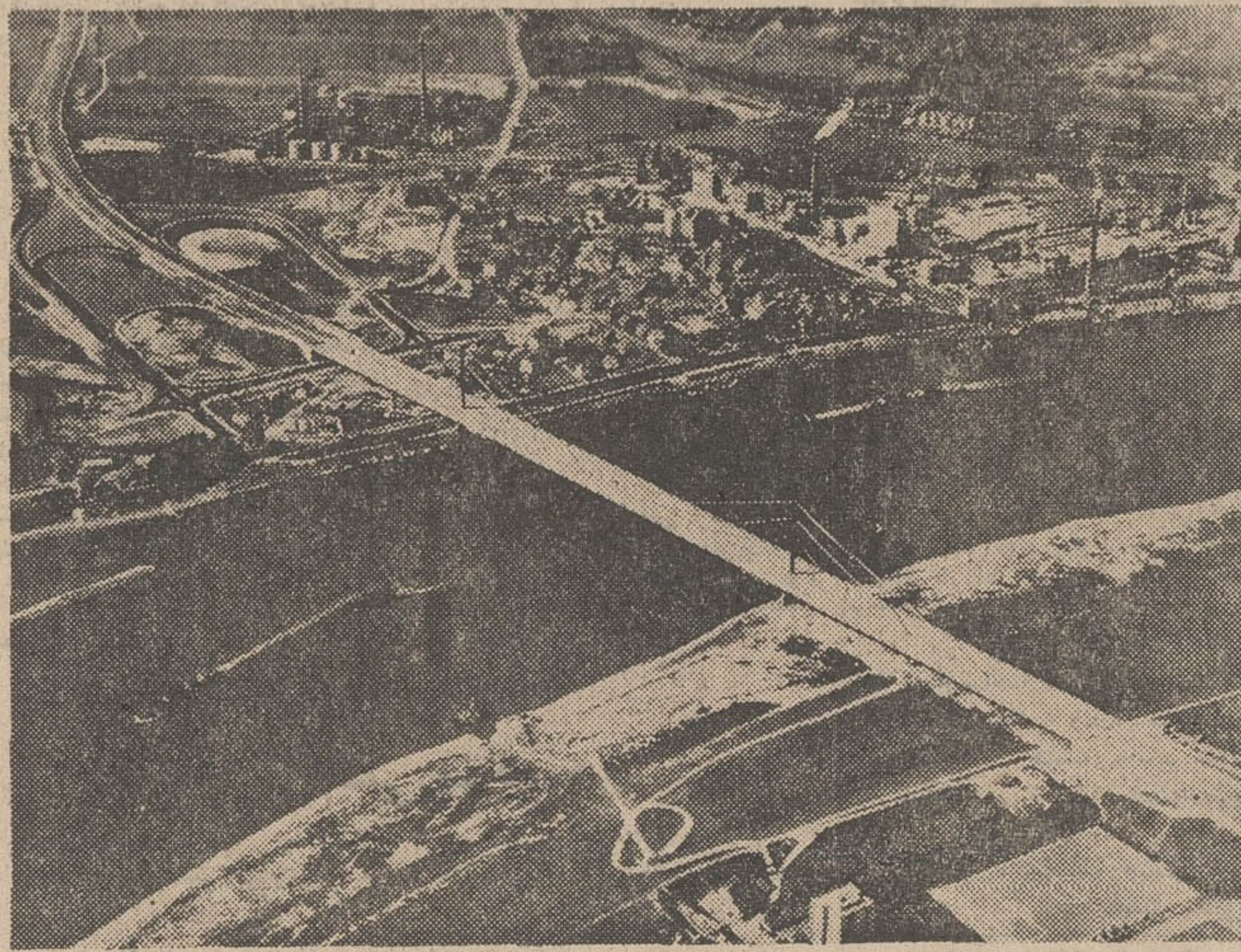
پل جدید در حوالی دوتزبورگ بروی رودخانه راین، از شاهکارهای صنعتی جهان نقلیه و عابران است. دهانه آن برای عبور کشتیها ۳۵۰ متر است.
