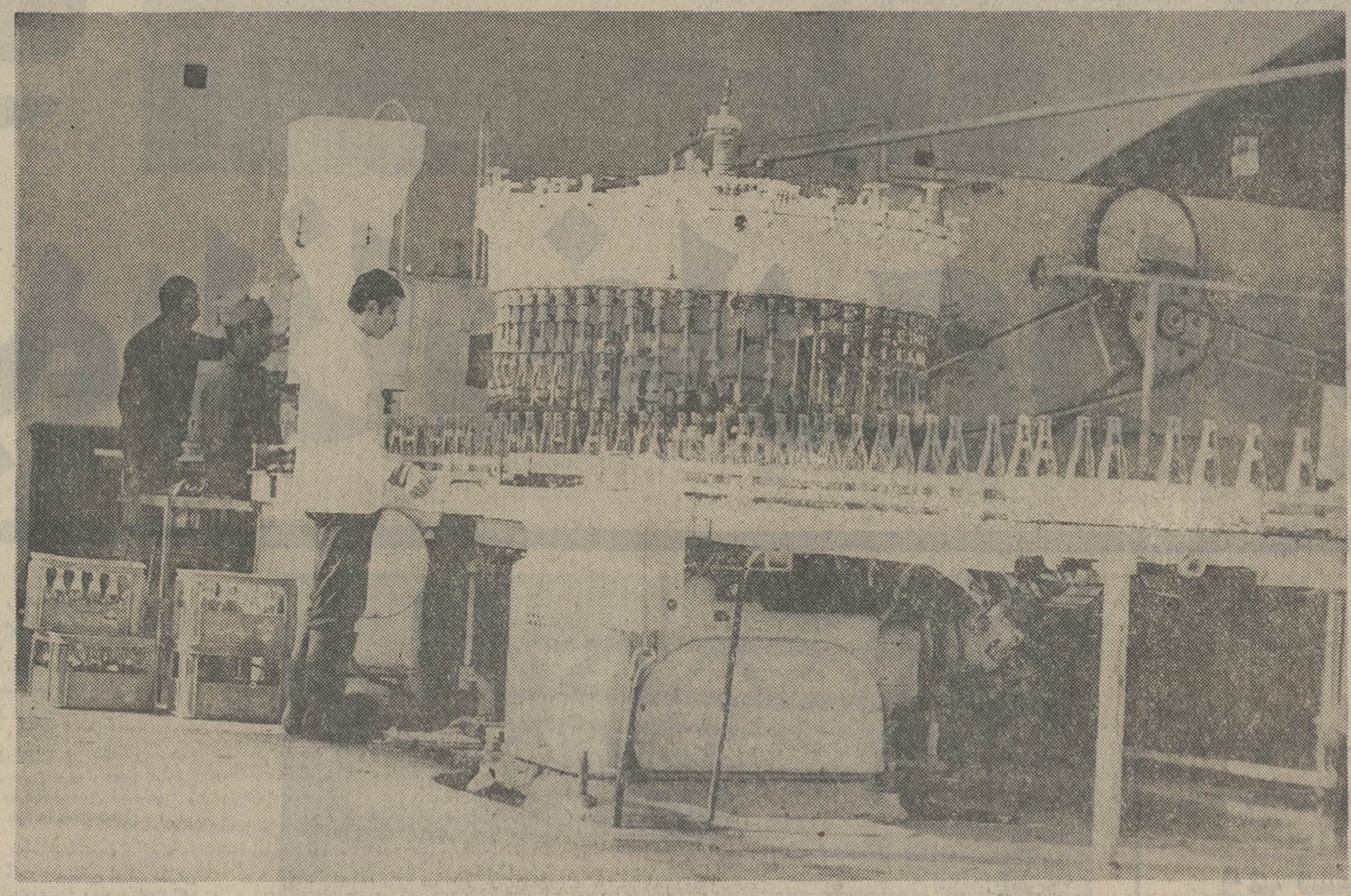
این نمائی از تاسیسات کارخانه دوغ آبعلی است که بدون دخالت دست، بطریهای خالی را پر از نوشابه کرده و بطور خودکار، در آنها را می بندد.
